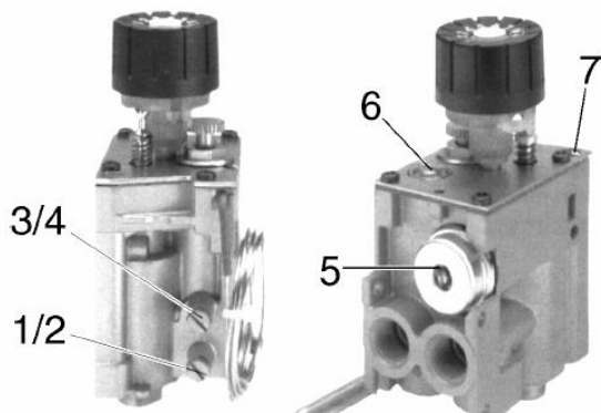
Sít-armatura Plynová armatura SIT
